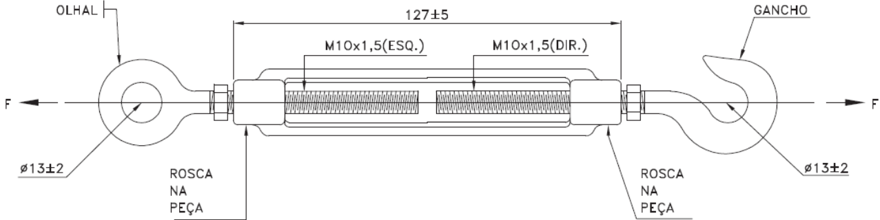
Figura 1 - Vista Lateral
