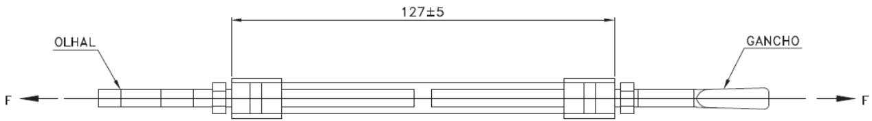
Figura 2 - Vista Superior
